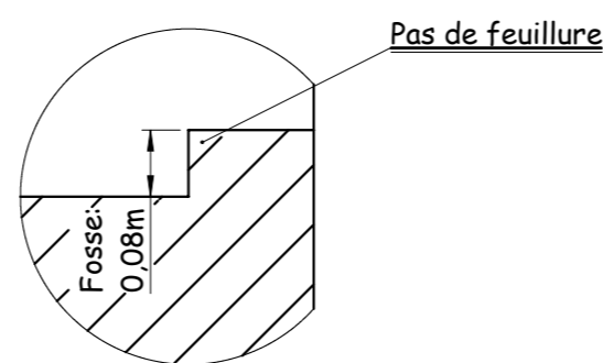
DÉTAIL a
